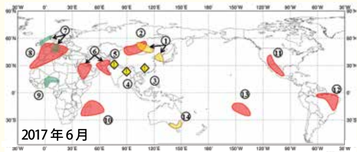
異常気象発生地域分布図 (気象庁)
