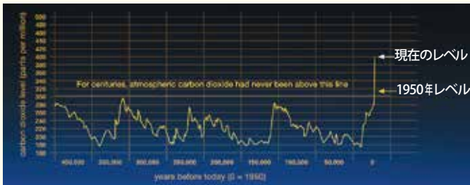
氷床コアに含まれた大気サンプル及び最近の直接的な測定によって、大気中のCO 2 が産業革命以後、いかに増えたかを示す表。
