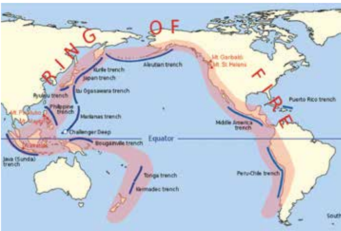
環太平洋火山帯
