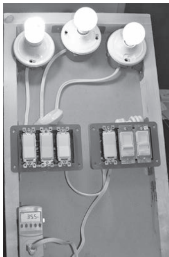
筆者作、ディマーと電球の簡易実験装置
